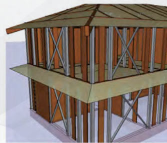
ASTIM/ 壁フレームによる軸組モデル
